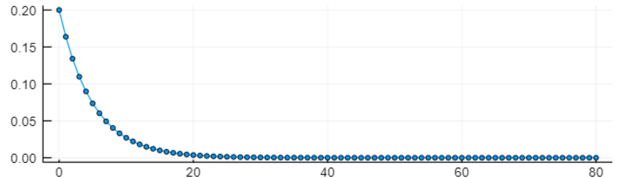
Eksponeñcijalna raspodela - gustina raspodele verovatnoc
